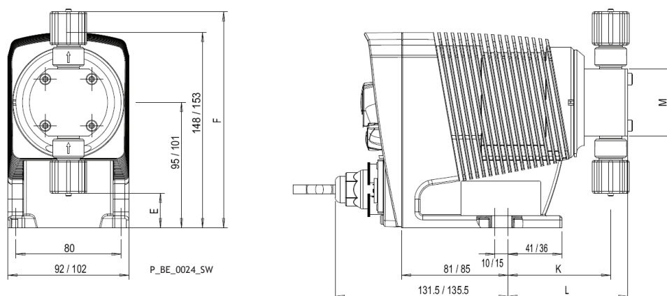
Рис. 18: Размерный чертеж Beta® BT4b/BT5b, Материал конструкции TT — размеры в мм
