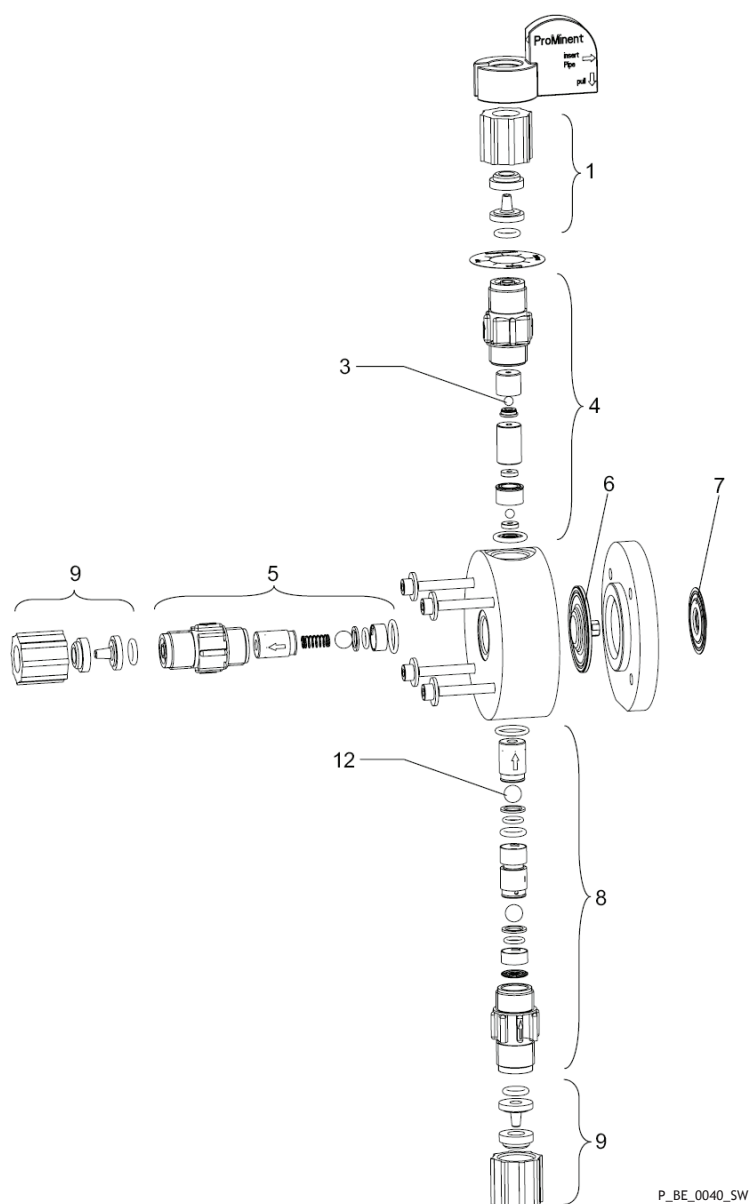
Рис. 40: Узел подачи Beta® 0708 (1008) - 0220 (0420) PP / NP SEK, с автоматической деаэрацией
