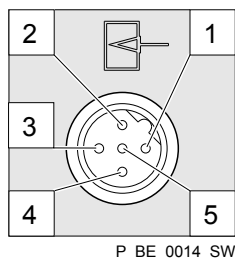
Рис. 11: Схема расположения контактов на насосе
