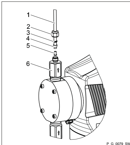
Рис. 9: Исполнения SS со шлангом
