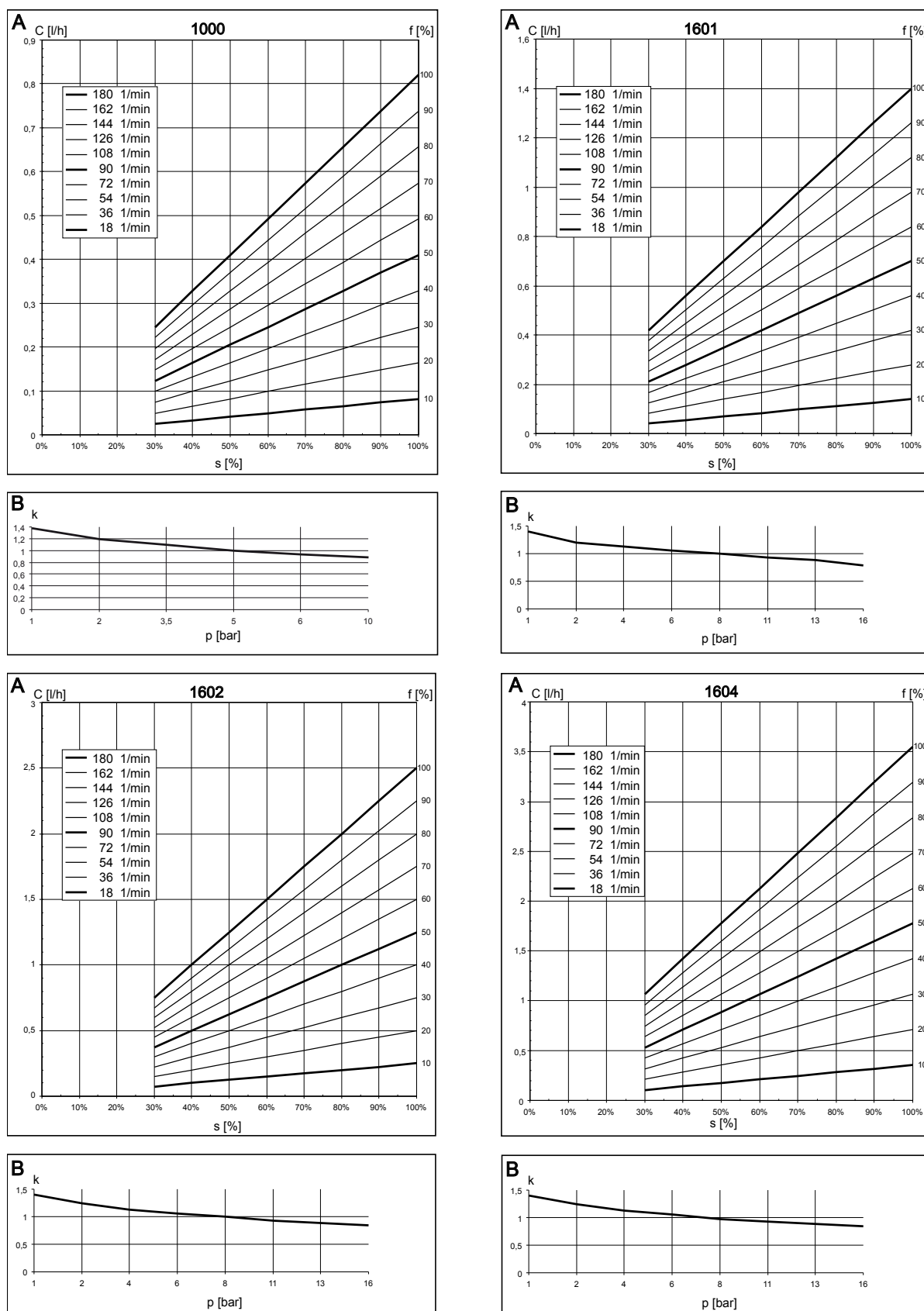
Рис. 59: А) Производительность дозатора C при среднем противодавлении в зависимости от длины хода s для различной частоты хода f . В) Соответствующие поправочные коэффициенты k в зависимости от противодавления p
