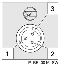
Рис. 13: Схема расположения контактов на насосе
